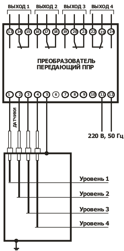
Рис. В.1 – Вариант для металлических резервуаров
