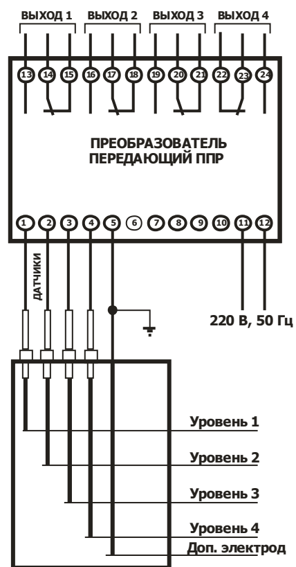
Рис. В.2 – Вариант для резервуаров из непроводящих материалов
