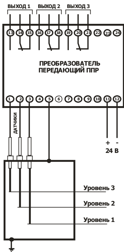
Рис. В1 – Вариант для металлических резервуаров
