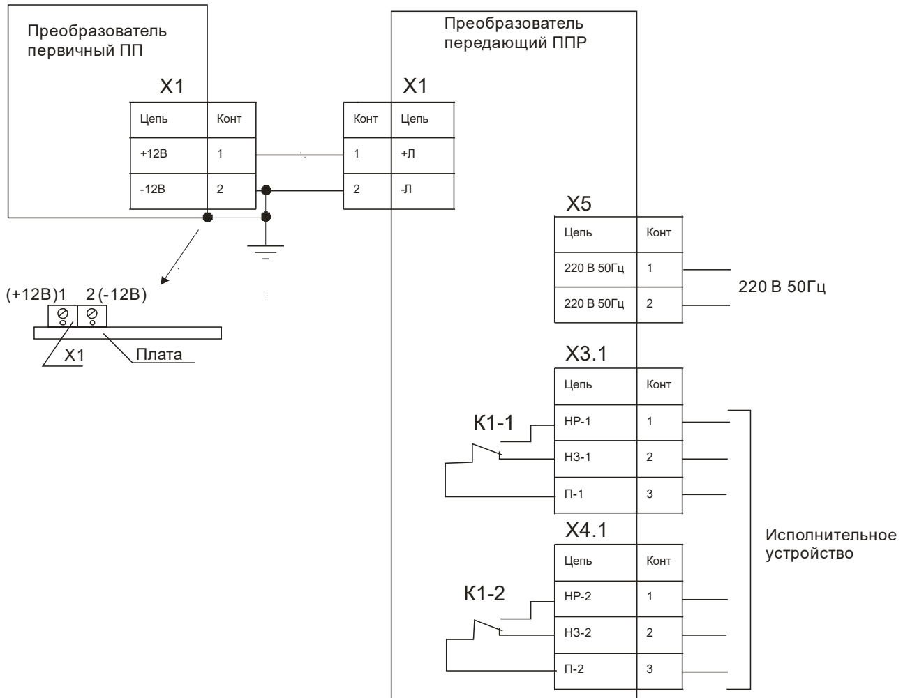
Рис. В.2 - Схема подключения ПРУ-5М (невзрывозащищенное исполнение)
