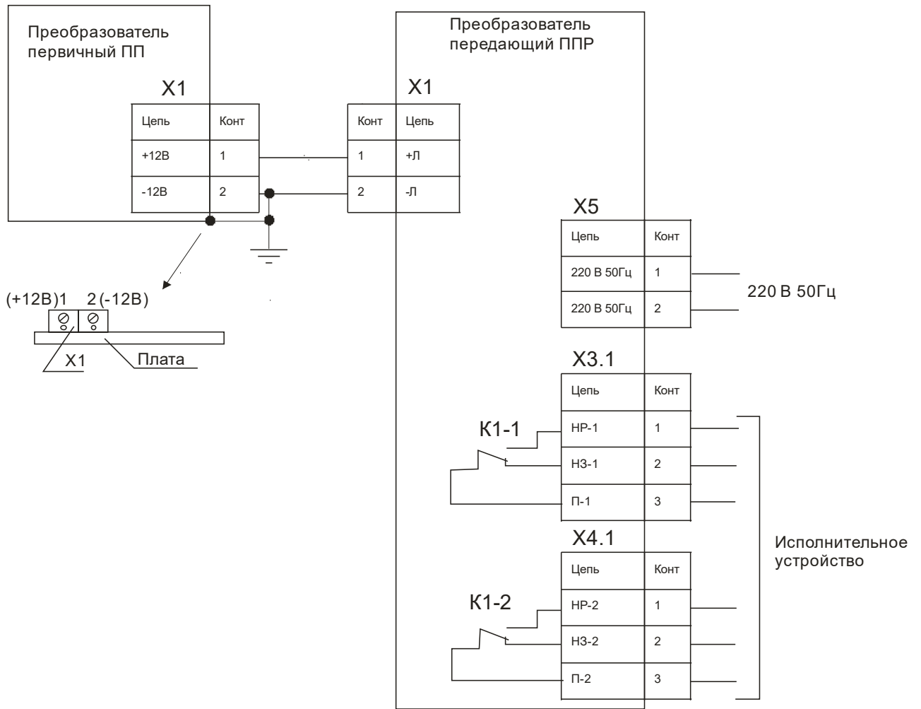
Рис. В.2 - Схема подключения РОС-501 (невзрывозащищенное исполнение)
