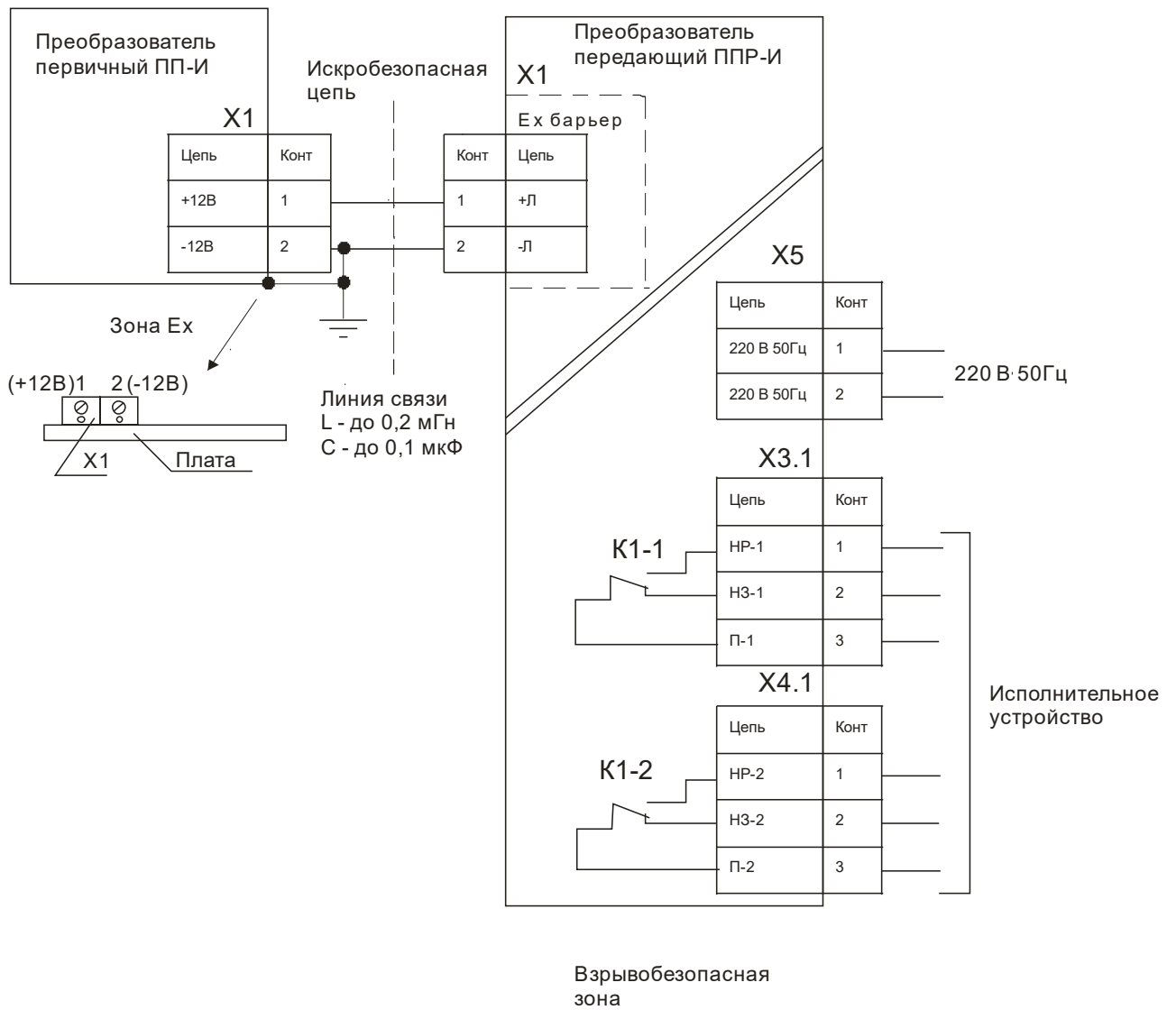
Рис. В.1 - Схема подключения РОС-501И (взрывозащищенное исполнение)
