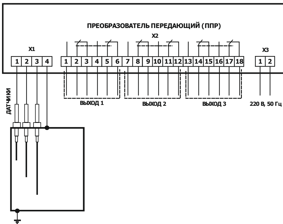
Рис. В.1 – Вариант для металлических резервуаров
